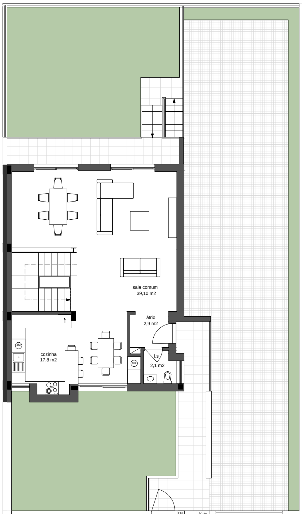
Planta do Lote02 Rês do Chão
