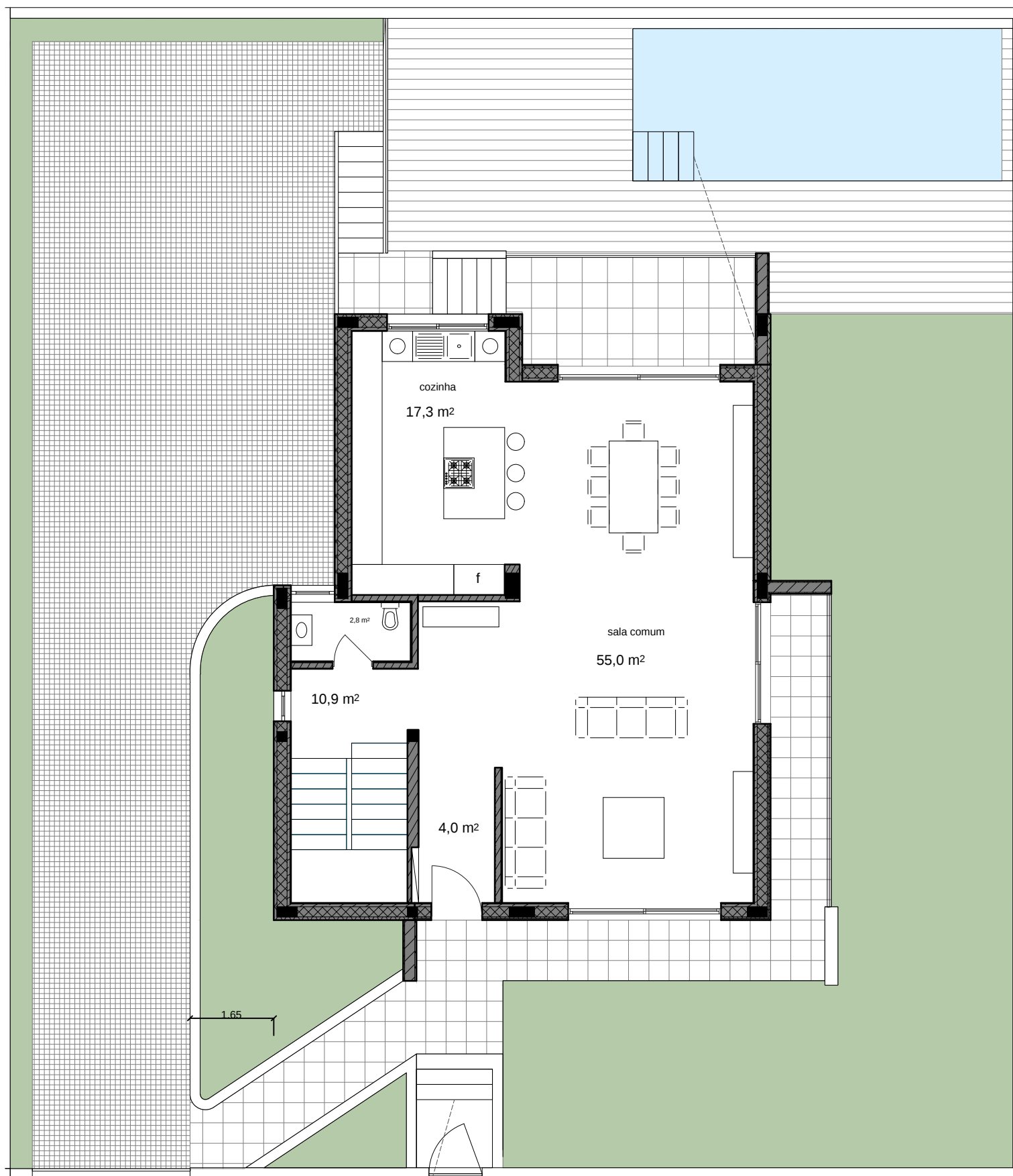
Planta do Lote03 Rés do Chão
